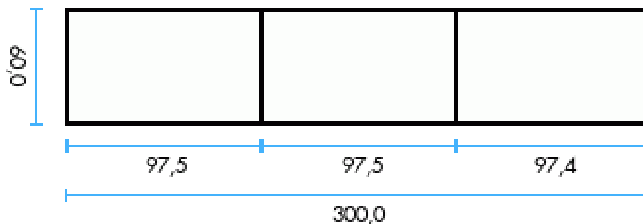
Draufsicht
